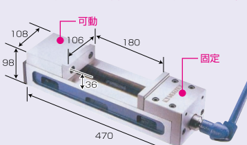
185 バーテックス マシンバイス (VCM-47) ●最大締付力: 450kgf ●質量:17.7kg ¥148,400
